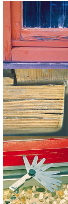
die abbildungen zeigen oberflächenrisse bei fenstern aus nadelholz
